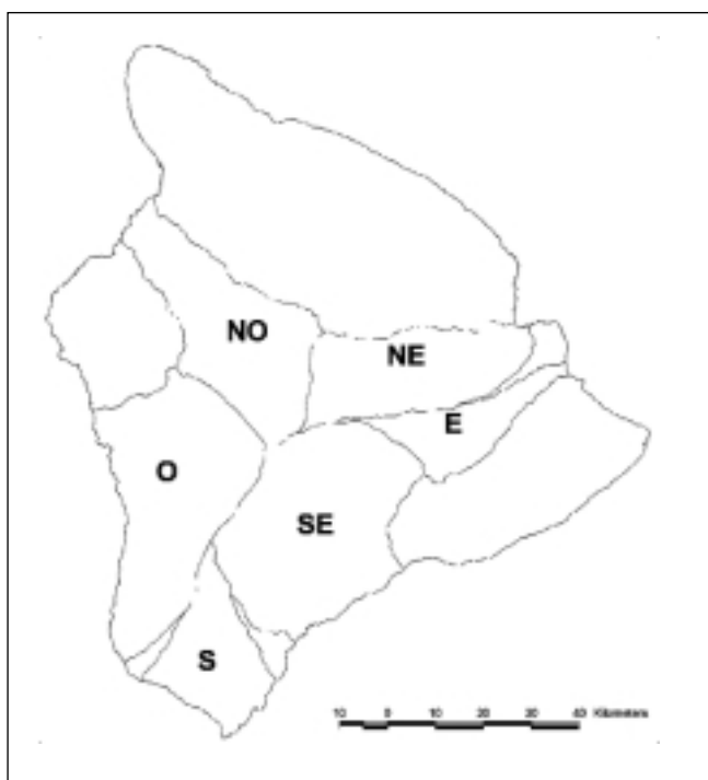
Figura 3. Regiones volcánicas.
